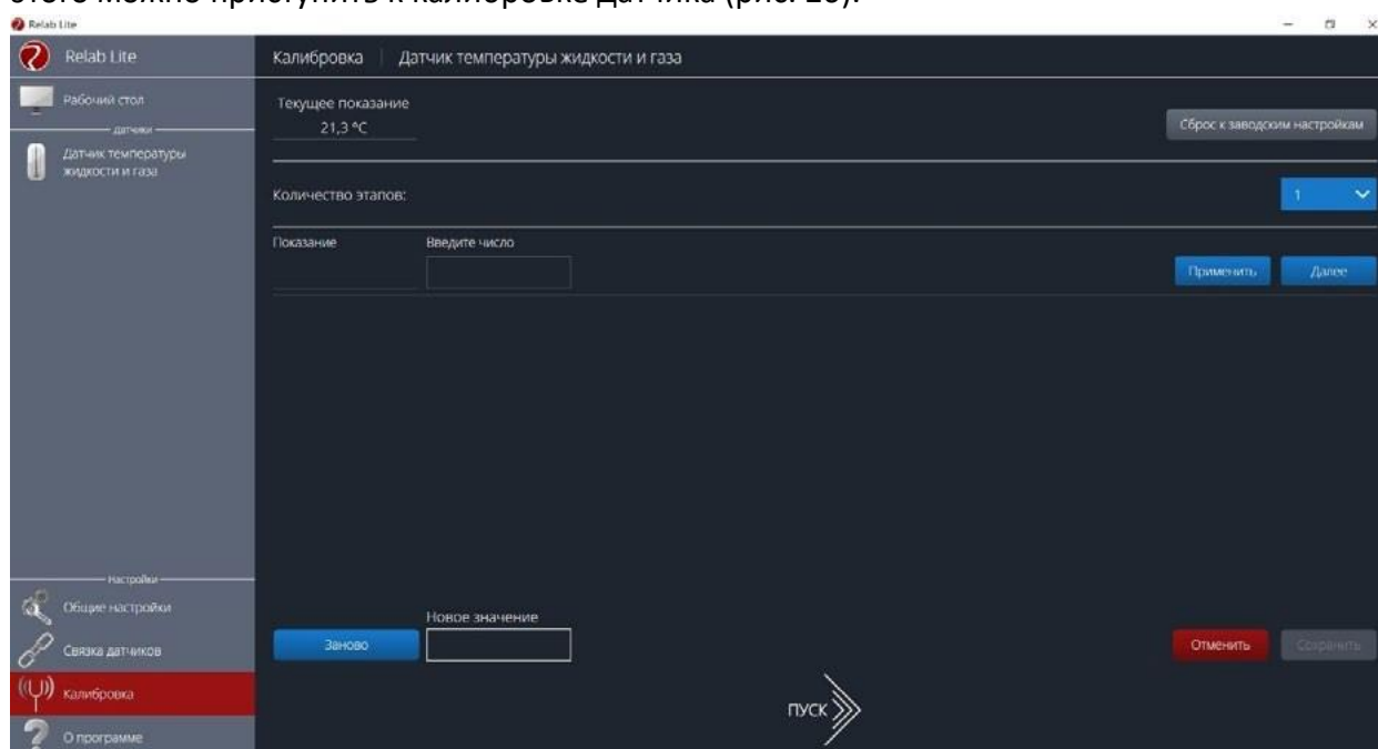
Рис. 26. Калибровка датчика
